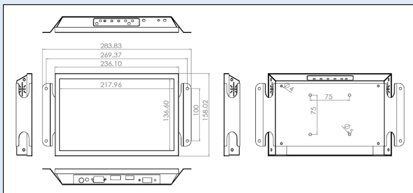
螢幕加 Open-frame 支架尺寸圖
