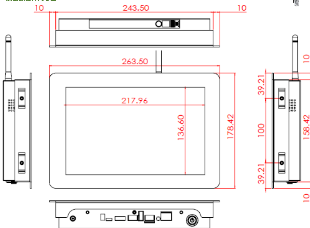
加前嵌套件尺寸圖
