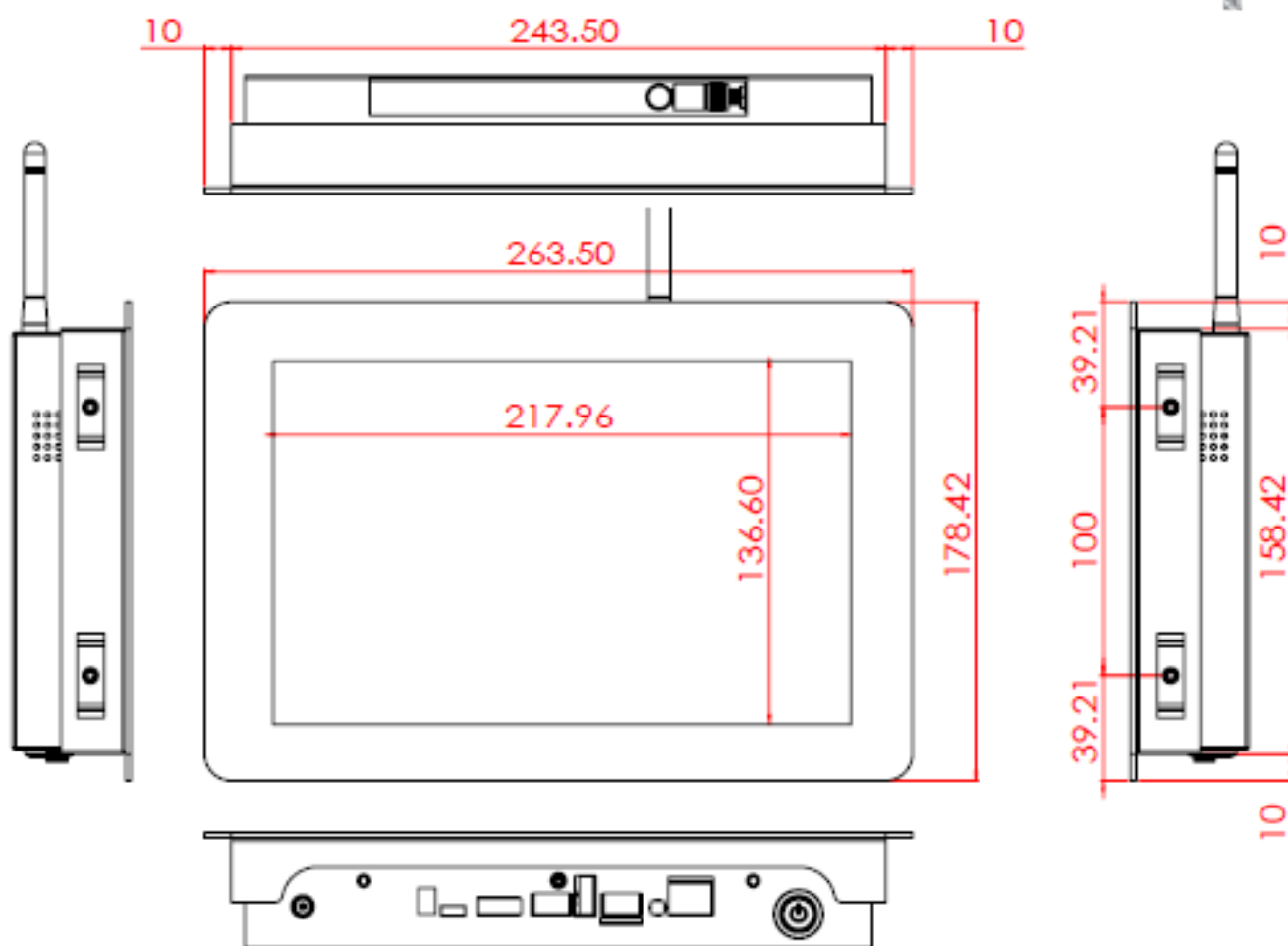
カバーフレームを取り付けの寸法
